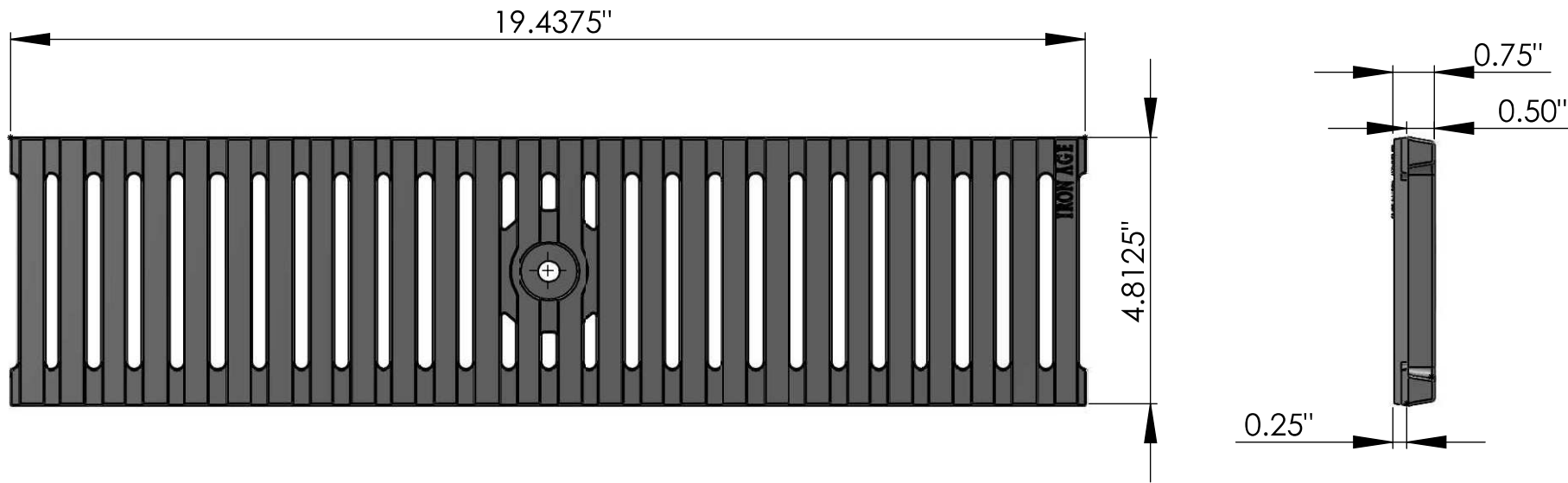
END scale 1:3
