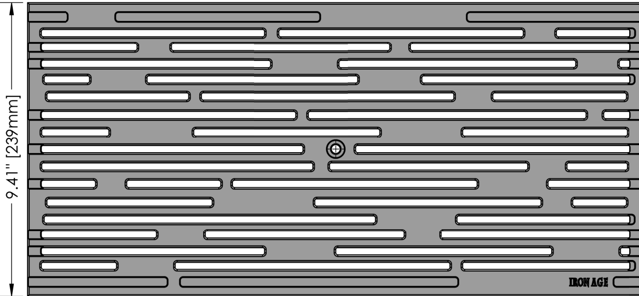
Top Scale 1:3
