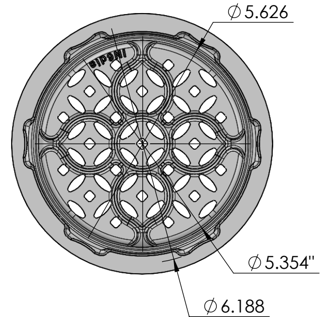
ISO-VIEW scale 1:3
