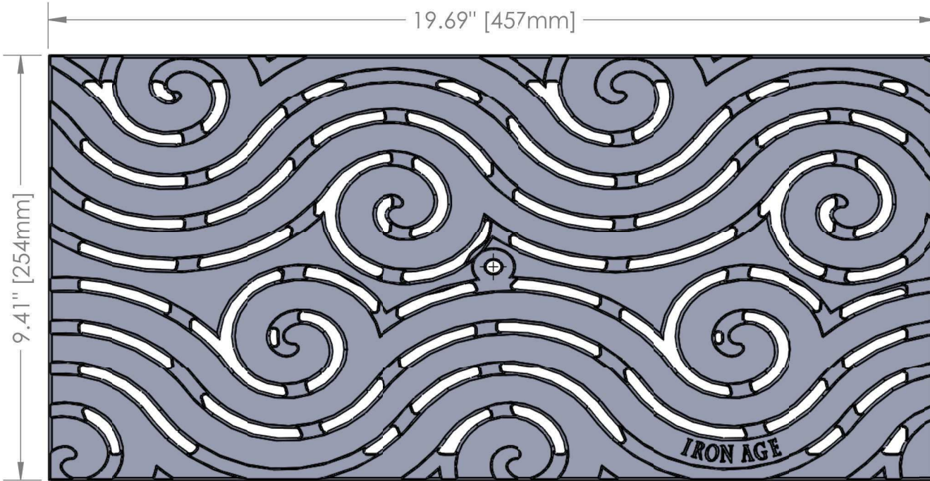
Top Scale 1:3
